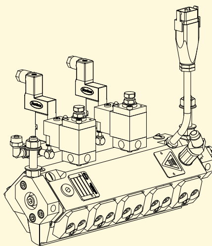
AltaSlot -c applicator
